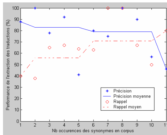
FIG. 5–Performance de la méthode en fonction du nombre d'occurrences des synonymes dans le corpus CISMeF/Hansard.
